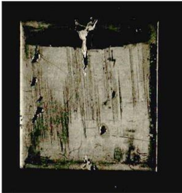
Afb. 3b. Zelfde-proefplaatje als foto 3a, andere zijde; hier treedt sterke spleetcorrosie en putvormige corrosie op. Deze zijde wordt gekenmerkt door veel mechanische oppervlaktebeschadigingen.
