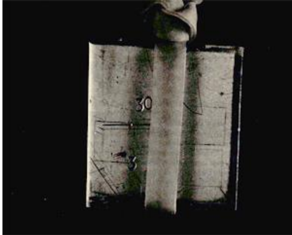
Afb. 2. Proefpleetje (rvs AISI 304), voorzien van elastiekje, voor onderdompeling in testoplossing (3% NaCl + 10% Fe 2 (SO 4 ) 3 in water).
