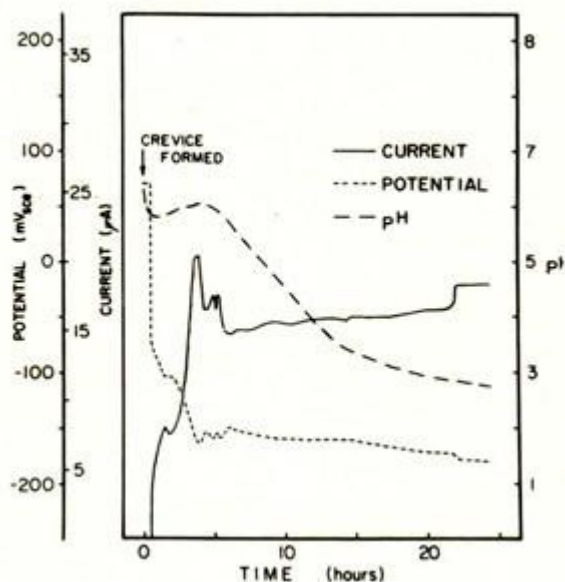
Afb. 7. Verloop van potentiaal, pH en corrosiestroom tijdens spleetcorrosie aan AISI 304, bij 55°C. [4]
