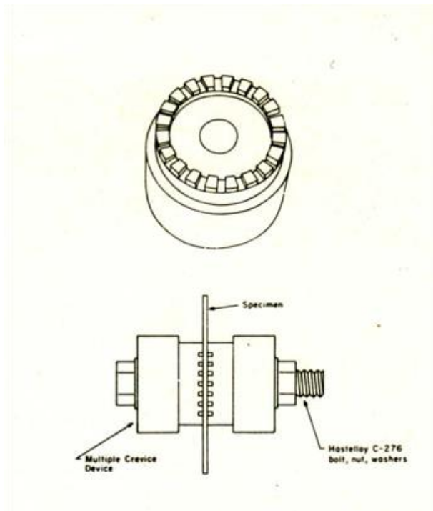
Afb. 5. Proefplaatje met gegroefde onderleggingen.
