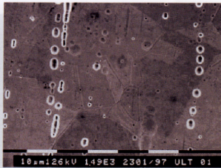
Afb. 3 Elektrolytisch gepolijst roestvast staal (316L). Het oppervlak vertoont geen kanaalvorming meer. V = 1500x
