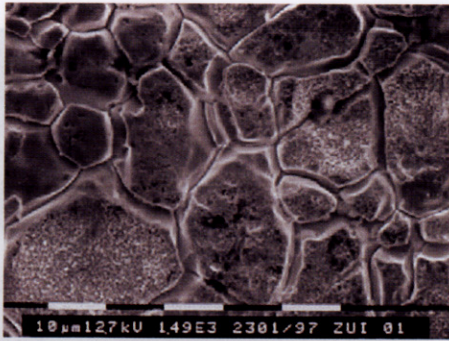
Afb. 2 Microscopische opname van een gebeitst roestvast staal (AISI 316L). Duidelijk is de kanaalvorming te zien op de korrelgrenzen. V = 1500x
