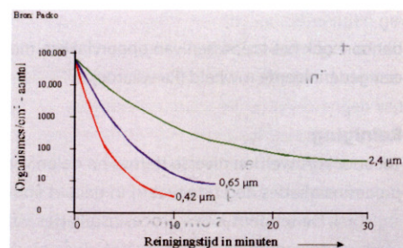
Afb. 5 De reinigingstijd als functie van de ruwheid van het staaloppervlak (bron: Packo België)
