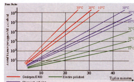
Afb. 4 Het effect van elektrolytisch gepolijst oppervlak met betrekking tot de afzet van vreemde deeltjes (bron: Packo België)
