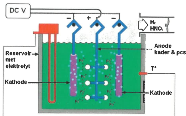
Het elektrolytisch polijstproces: de metaalionen (het ijzer) van het te behandelen onderdeel worden verwijderd en aangetrokken tot de kathode
